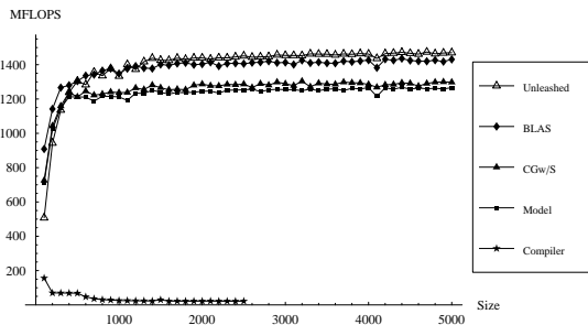
Fig. 12(d). DEC Alpha 21264: MMM Performance
